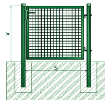
Š - Šírka medzi stĺpikmi
